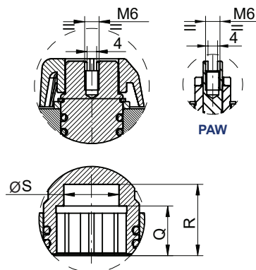
DETAIL HŘÍDELE
