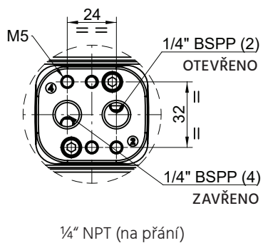
PLATFORMA PNEUMATICKÉHO PŘIPOJENÍ NORMA NAMUR E.V.
