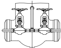
С уравновешивающей трубкой и байпасным трубопроводом
