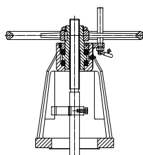
uzamykáč zařízení
