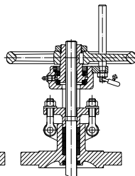
uzamykací zařízení
